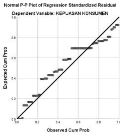
Gambar 2 Hasil Uji Normalitas Normal P-Plot
