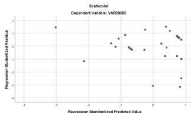
Gambar 3 Hasil Pengujian Heteroskedestisitas
